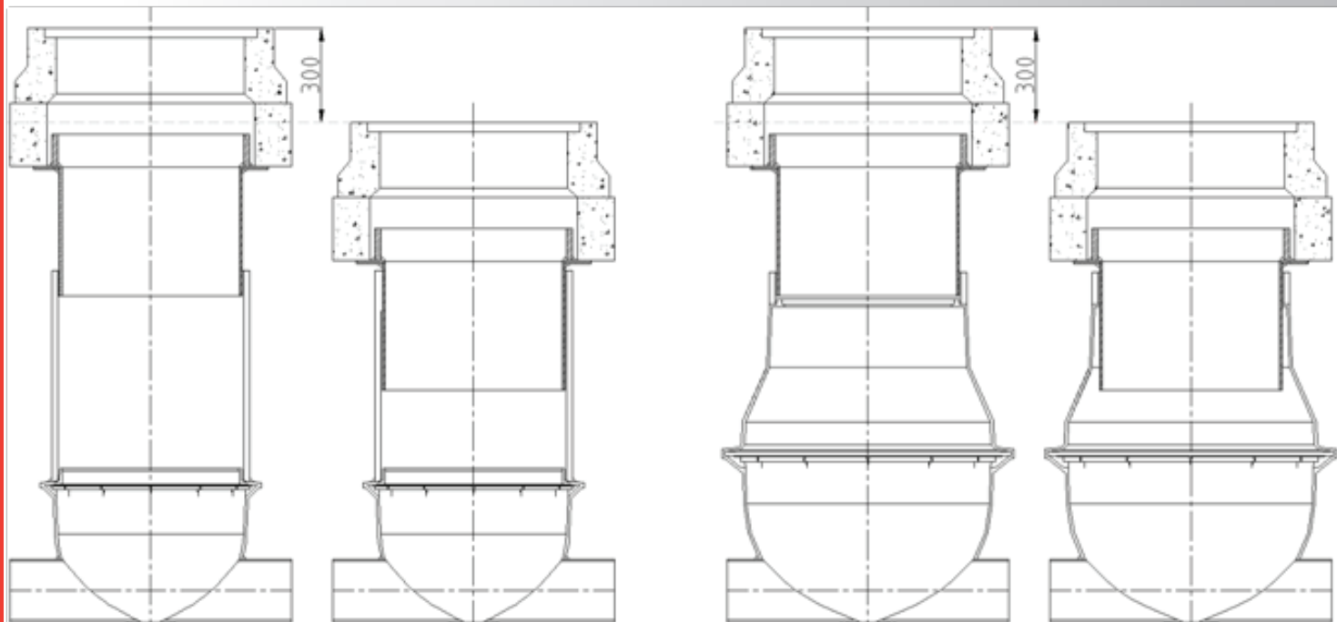
Enkele varianten bolle bodemputten die Beutech levert. Links de Ø630 mm met telescoopdeel in- en uitgeschoven, rechts de Ø800 mm met telescoopdeel in- en uitgeschoven.
